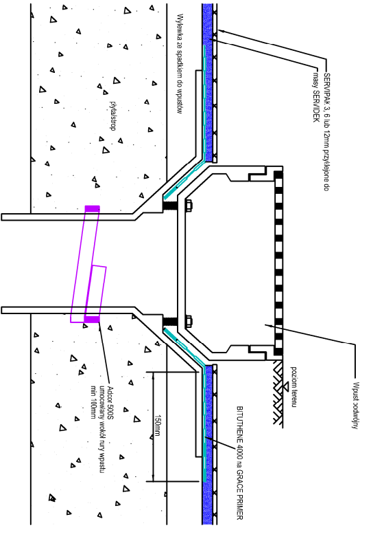
WPUST PODMÓWNY SERVIDEK / SERVIPAK PRZEKRÓJ
